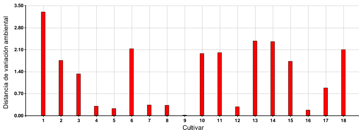
Figura 2: Diferencias de la distancia entre los índices de estabilidad multiambiental y la línea media Santa María Cahabón, Alta Verapaz, Guatemala 2019
